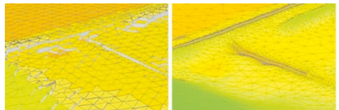
Abbildung 7: Beispiele für Finite-Volumen-Modelle (FVM). Links: auf Basis waagrecht triangulierter Elemente (Informationen und Berechnung auf den Elementflächen) und rechts: auf Basis geneigter Elemente (Informationen und Berechnung an den Knotenpunkten) (Quelle: Ruiz Rodriguez + Zeisler + Blank GbR)
